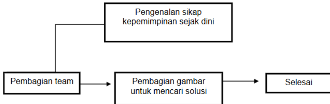
Gambar 1. Alur Aktivitas
